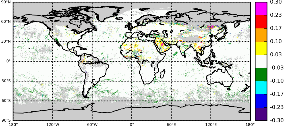
MODC OBS: TOP minus MIDDLE
