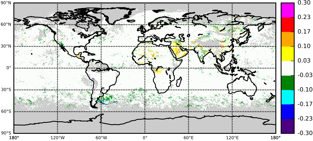
MODC OBS: TOP minus MIDDLE
