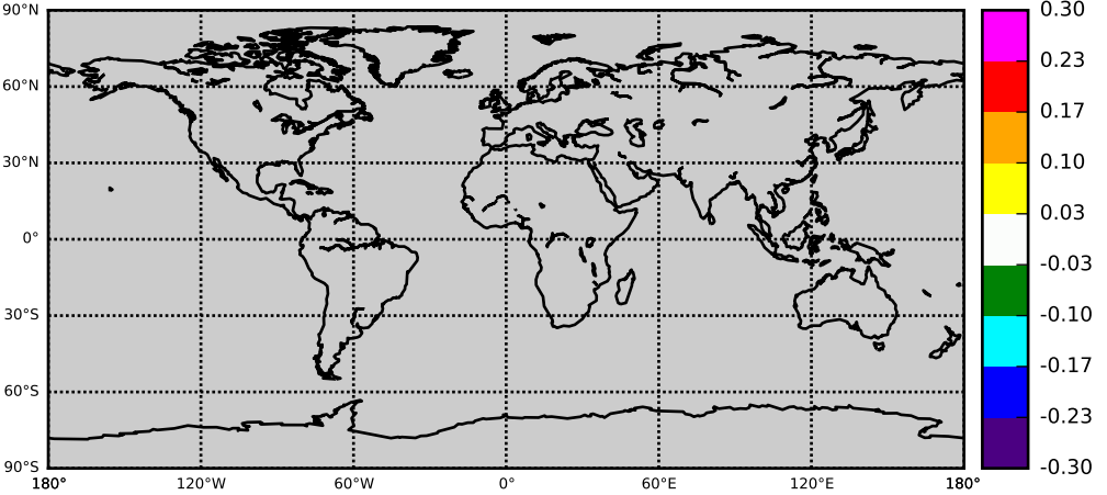
MYDD OBS: TOP minus MIDDLE
